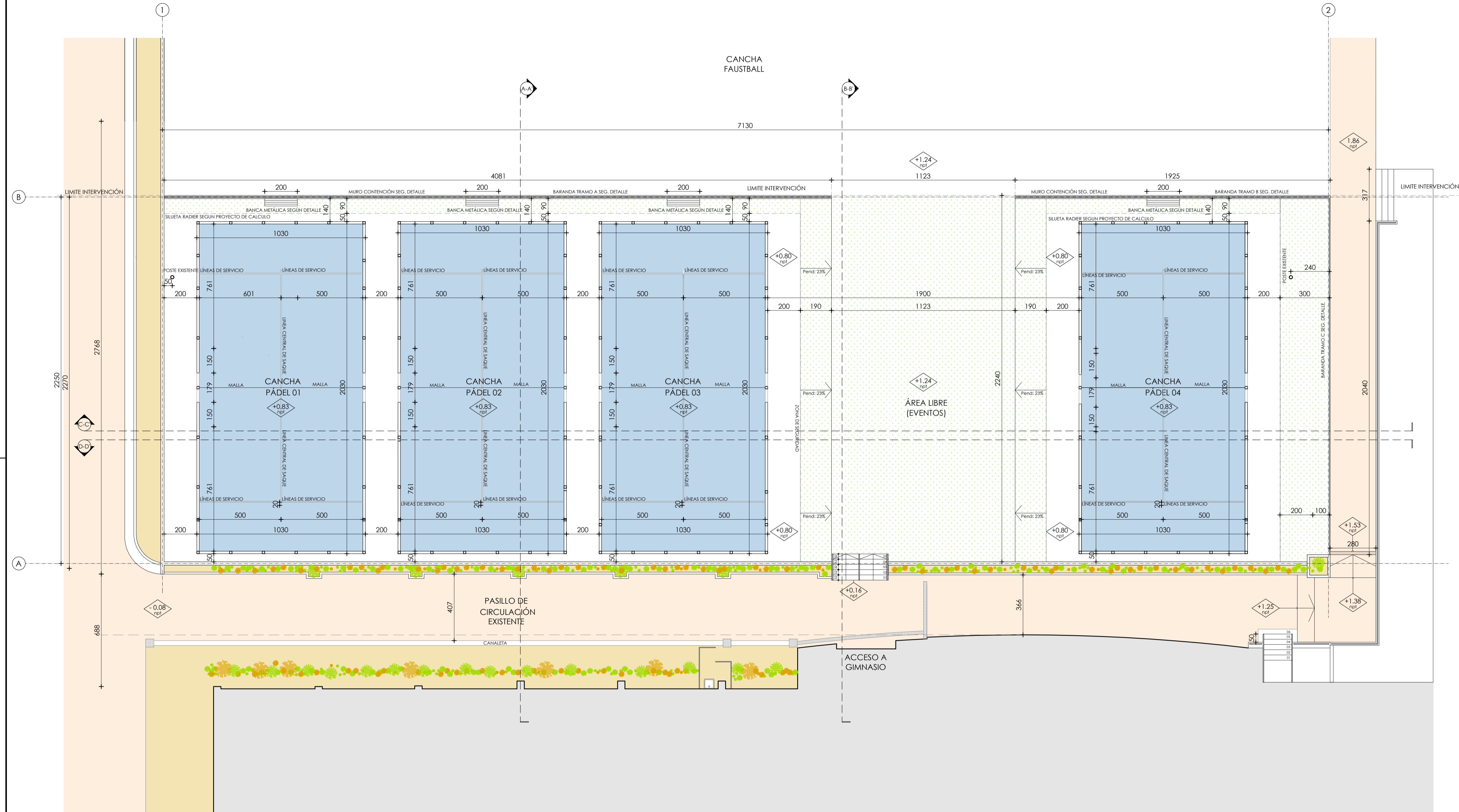
PLANTA DE ARQUITECTURA PROPUESTA escala 1/125
